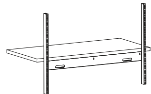
Kabelkanal zwischen Säulen Nutzhöhe 70 mm, für Steckdosenleiste (siehe Seite 95)
