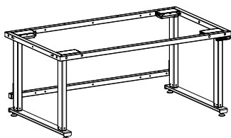
ERGO-Master, Grundgestell mit Elektromotor, höhenverstellbar von 730 – 1230 mm, Flächenbelastung 350 kg
