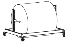
Abrollbock fahrbar bis Rollendurchmesser 750 mm und 150 kg, 4 Lenkrollen Ø 125 mm, davon 2 Stk. gebremst
