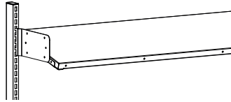
Ablageboden schwer mit verschraubter Konsole Neigung 0° und 15°, Tragkraft 50 kg
