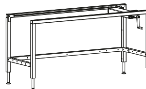
ERGO-Basic, Grundgestell verkürzt mit Handkurbel höhenverstellbar mit Handkurbel von 605 – 905 mm, Flächenbelastung max. 350 kg
