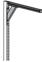
Ausleger komplett inkl. 30/30 Aluprofil Länge 670 mm
